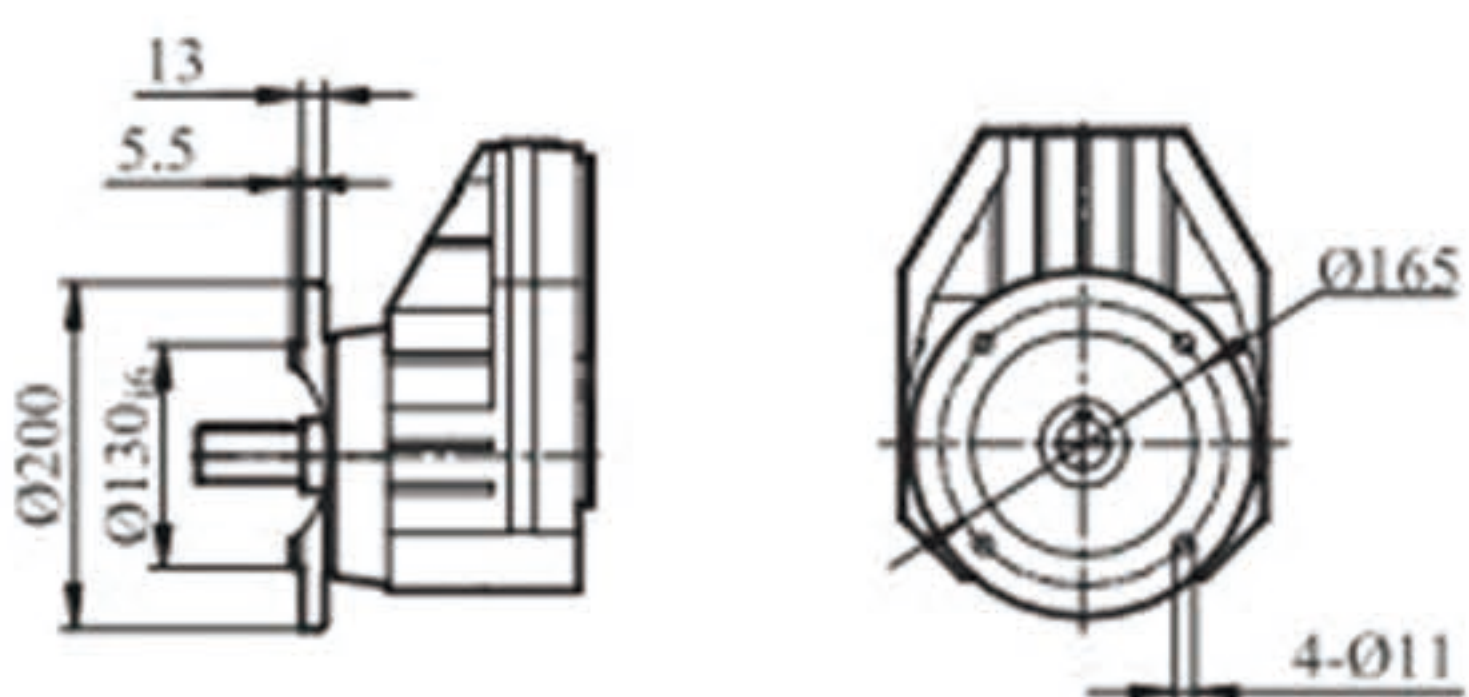
Ø200
