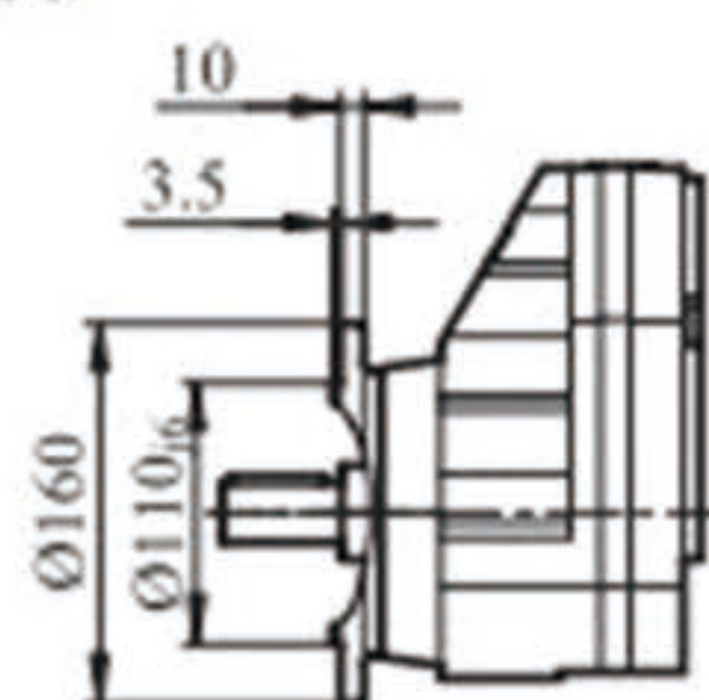
Ø160
