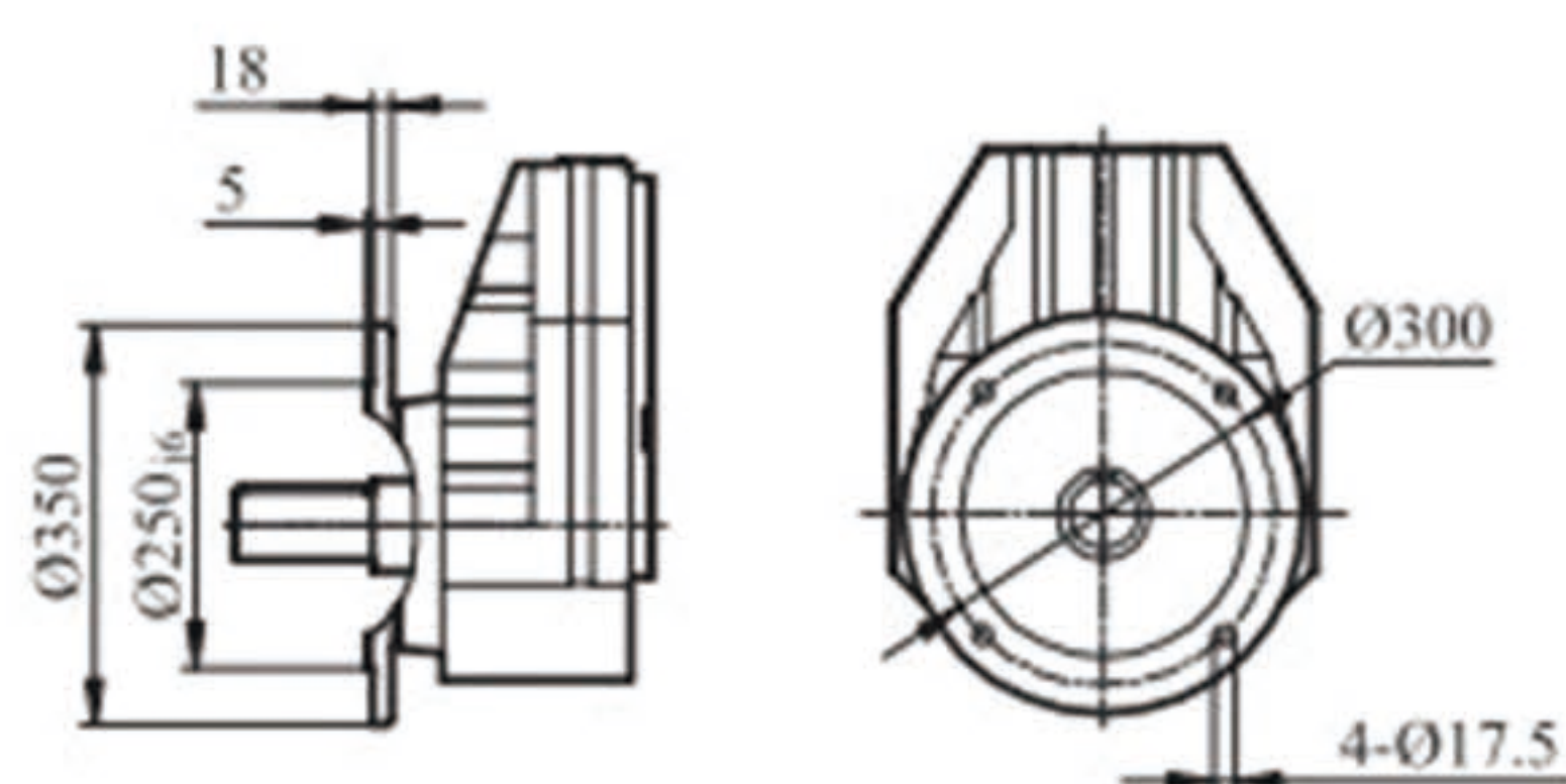
Ø350
