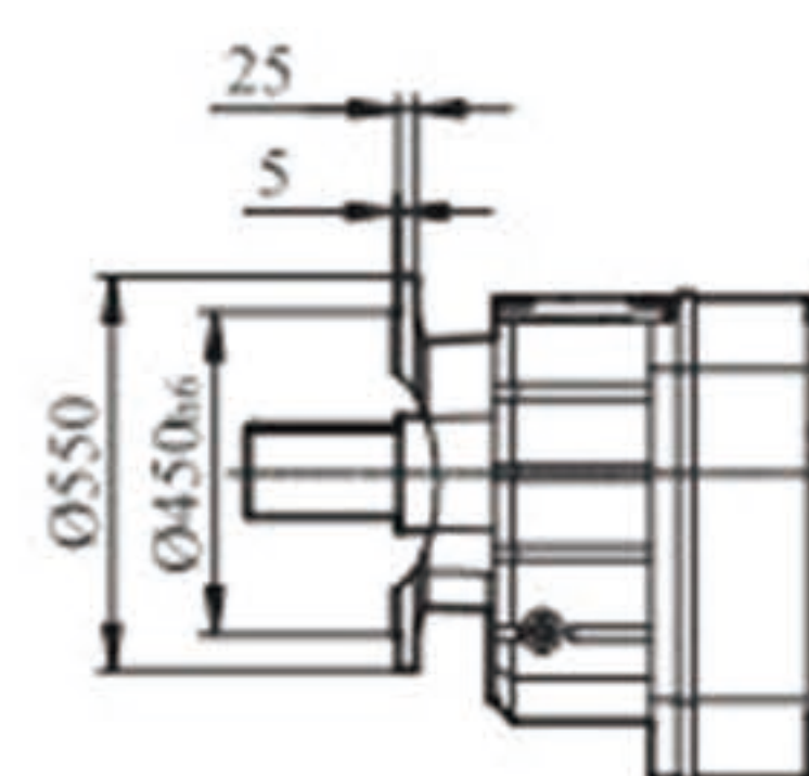
Ø550
